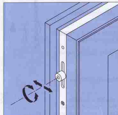
Flügelandruck regulieren
