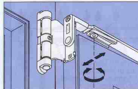
Flügelndruck einstellen
